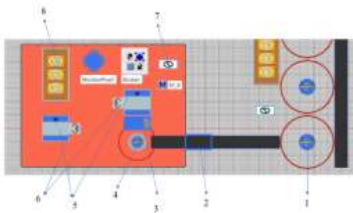
Hình 14. Khu vực kho lưu trữ. (1) robot vận chuyển, (2) băng tải nâng, (3) hệ thống tự động dán phiếu ngày nhập kho, (4) robot vận chuyển lên, (5) máy dán tem và máy kiểm tra ngày nhập kho, (6) vị trí di chuyển của công nhân trong khu vực kiểm tra sản phẩm vào kho, (7) hệ thống giám sát tổng sản phẩm lưu kho, (8) kho chứa hàng thành phẩm
