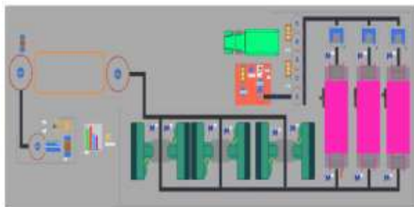
Hình 18. Tổng quan nhà máy sản xuất khay đựng bia và đóng gói bia tự động
